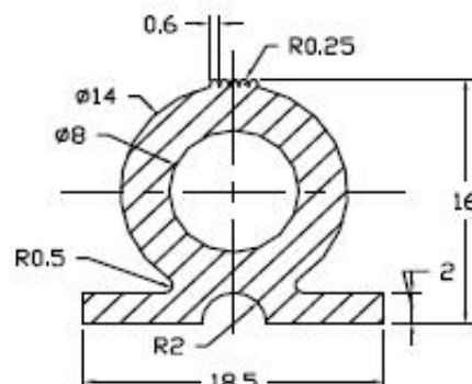
Profil : 5879
