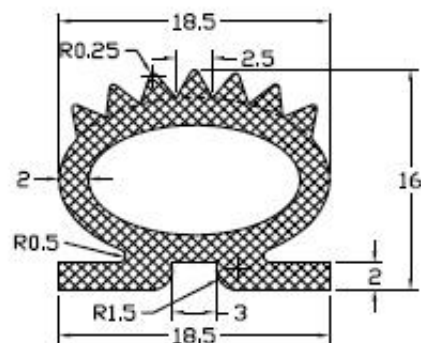
Profil : 5879
